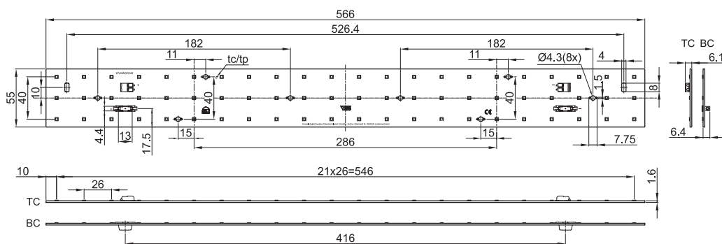
WU-M-536-S-TC/-BC
